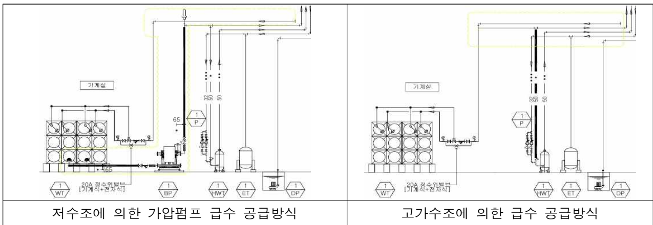
【표2】 급수 공급방식 변경 계통도
