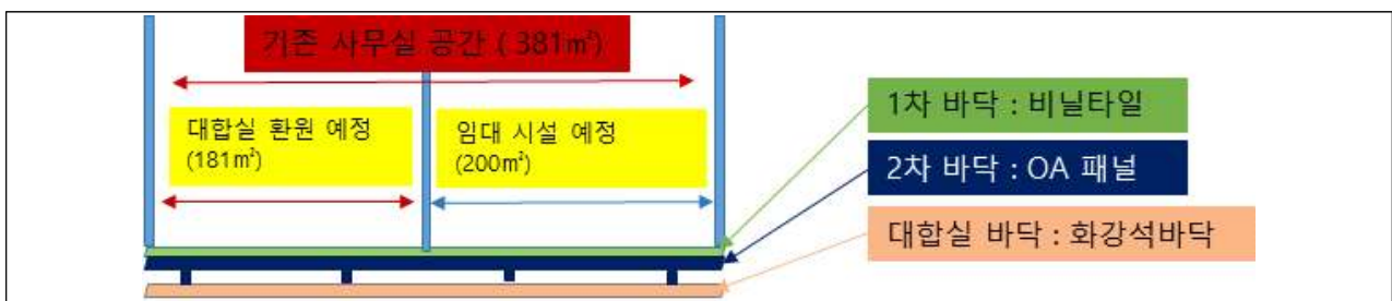
【표】 터미널 내부 리모델링 공사 바닥면 단면도
